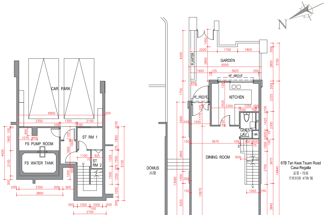
Basement Plan 地庫平面圖
