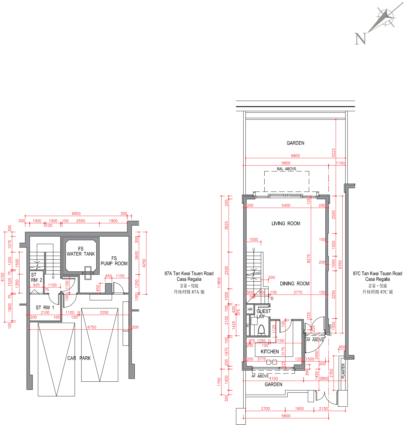
Basement Plan 地庫平面圖
