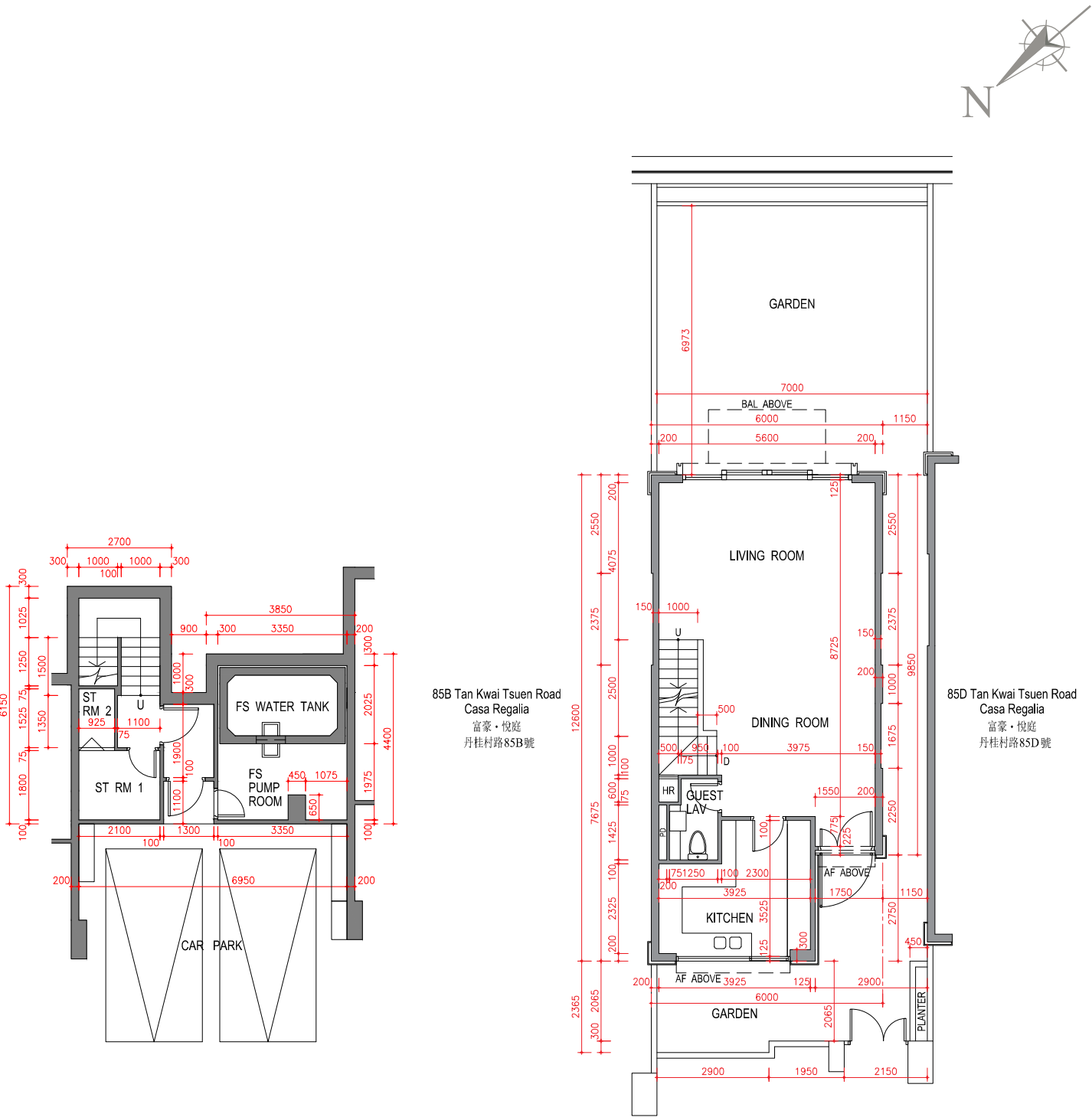
Basement Plan 地庫平面圖
