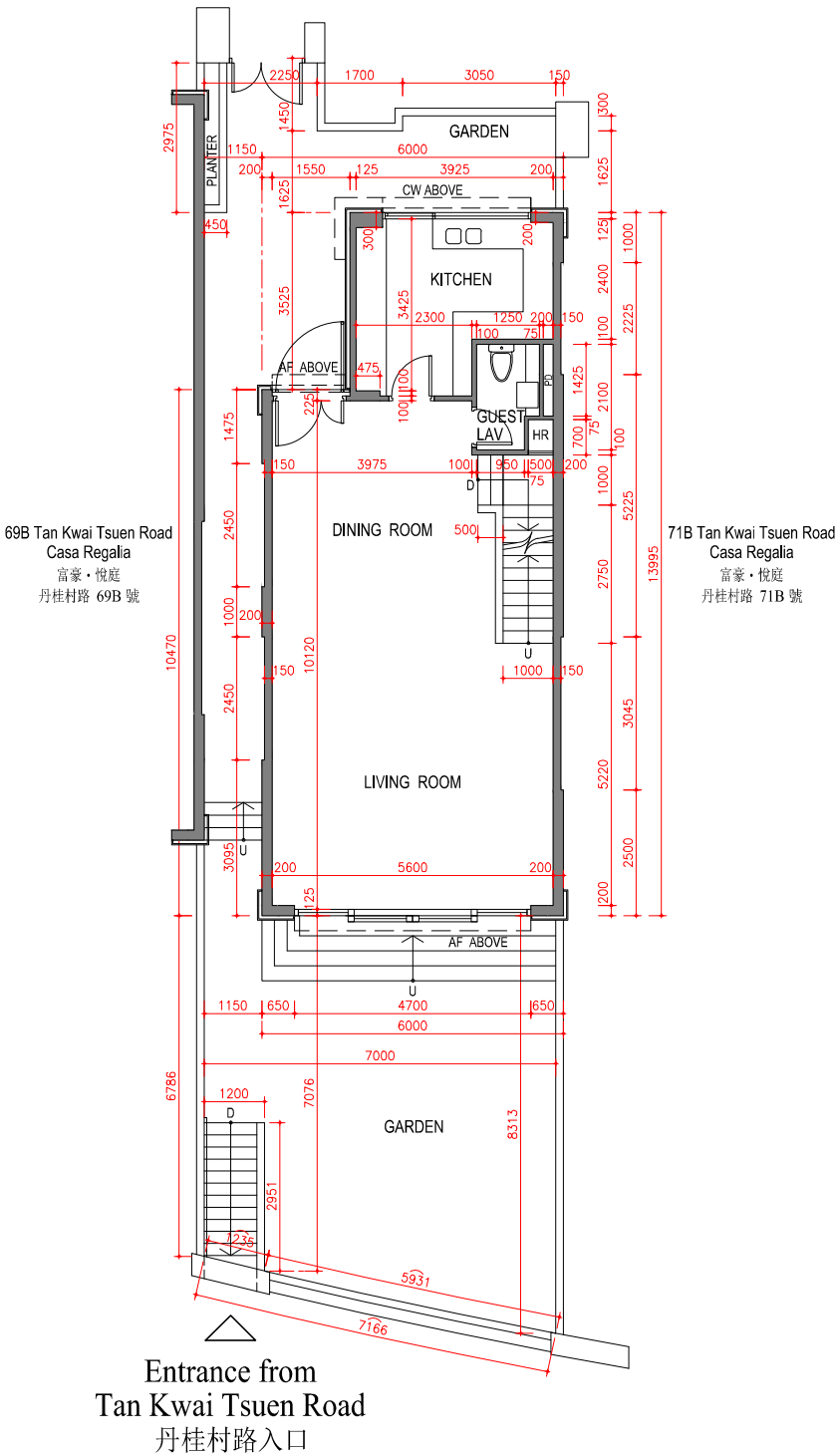
G/F Plan 地面層平面圖
