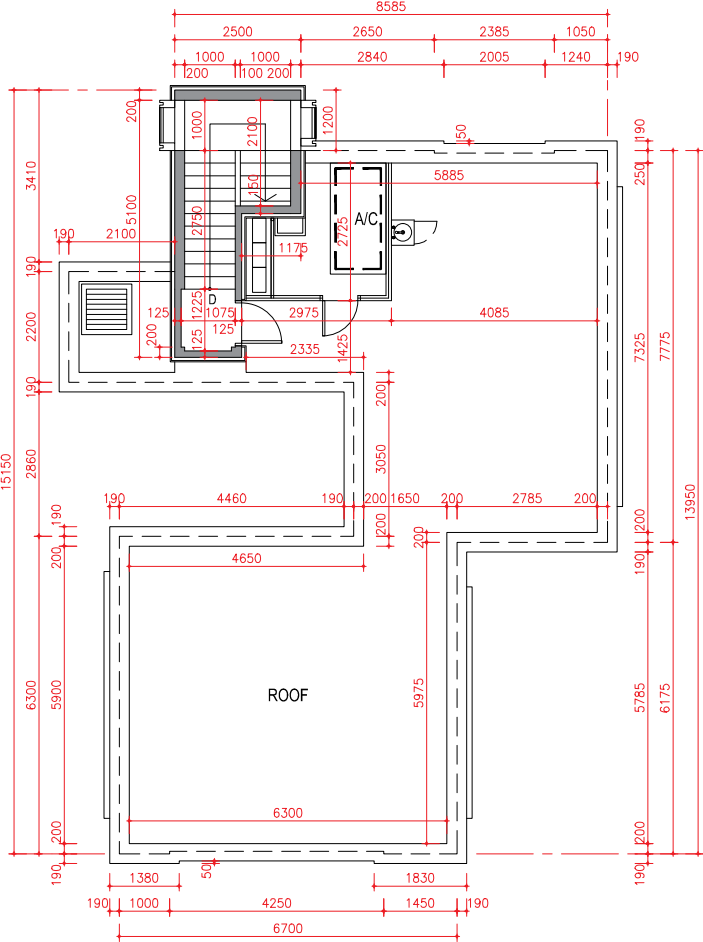
Roof Plan 天台平面圖
