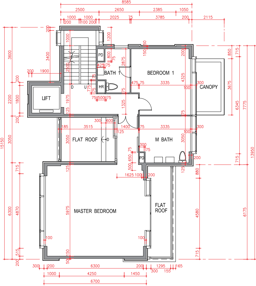
2/F Plan 二樓平面圖
