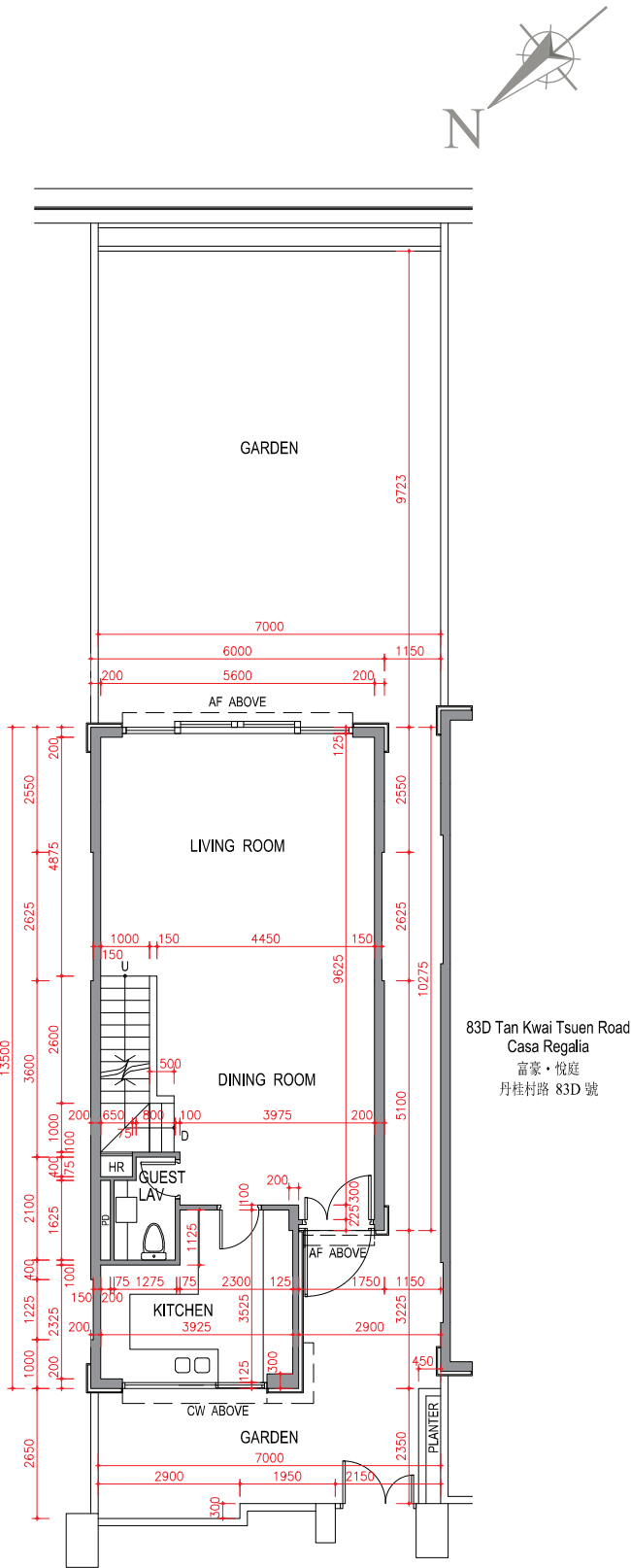
G/F Plan 地面層平面圖
