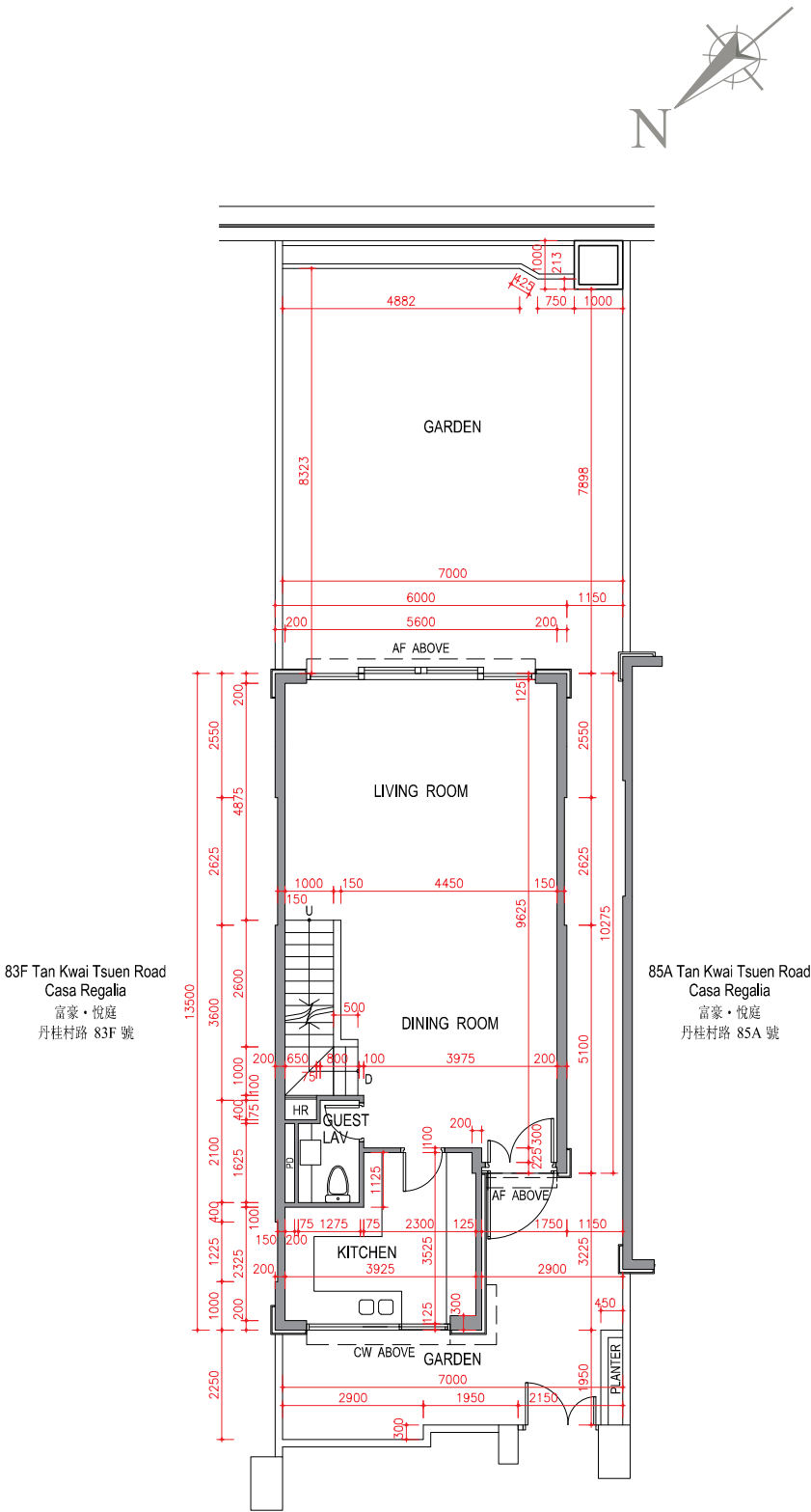
G/F Plan 地面層平面圖
