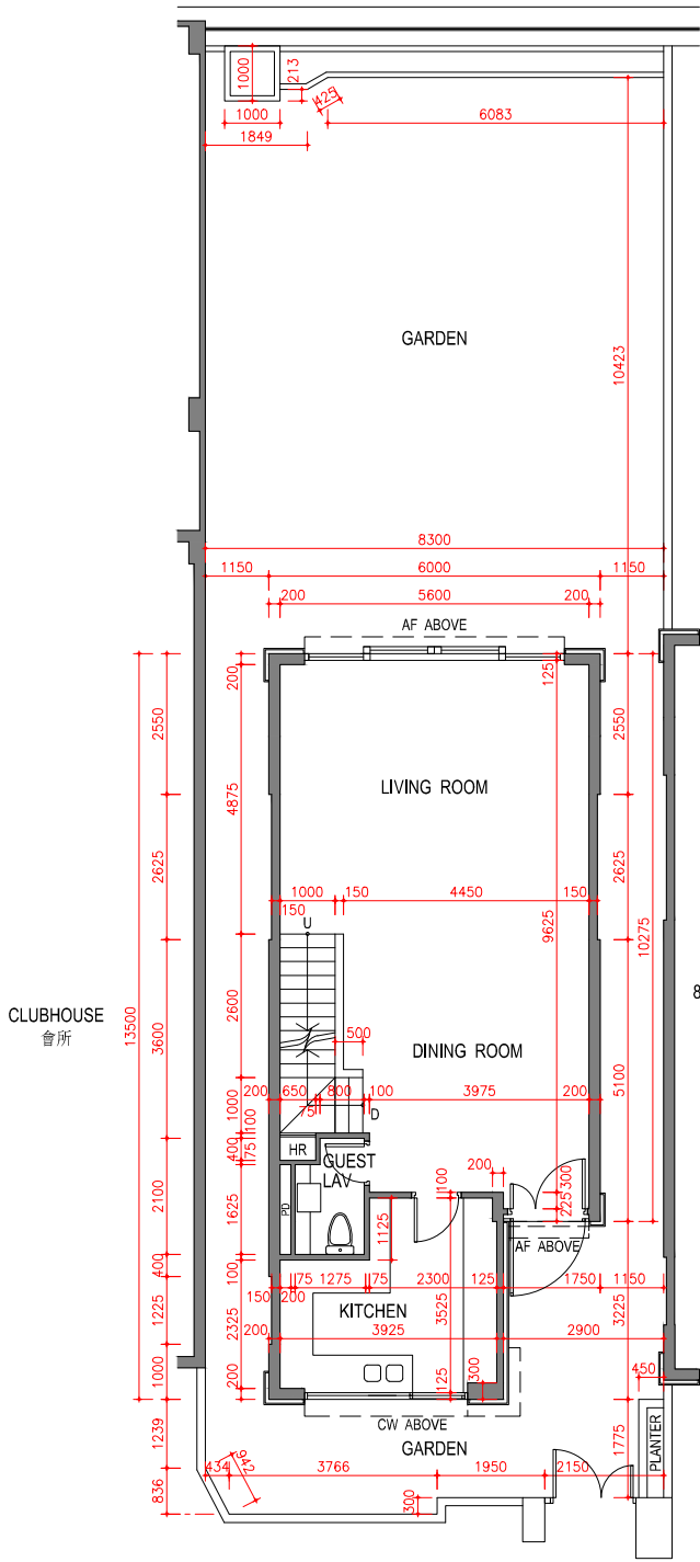
G/F Plan 地面層平面圖
