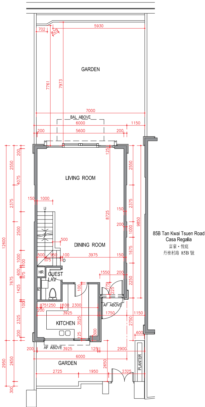
G/F Plan 地面層平面圖
