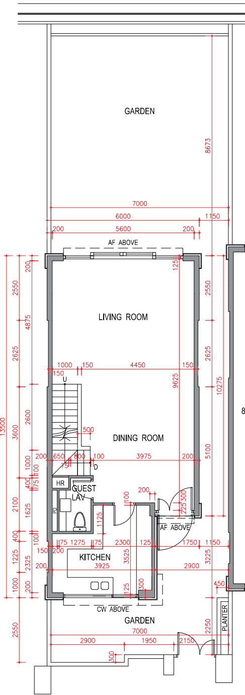
G/F Plan 地面層平面圖
