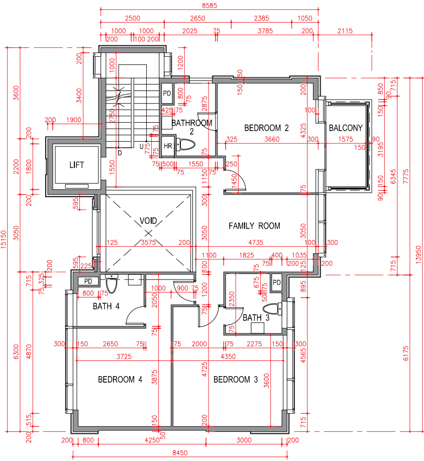
1/F Plan 一樓平面圖
