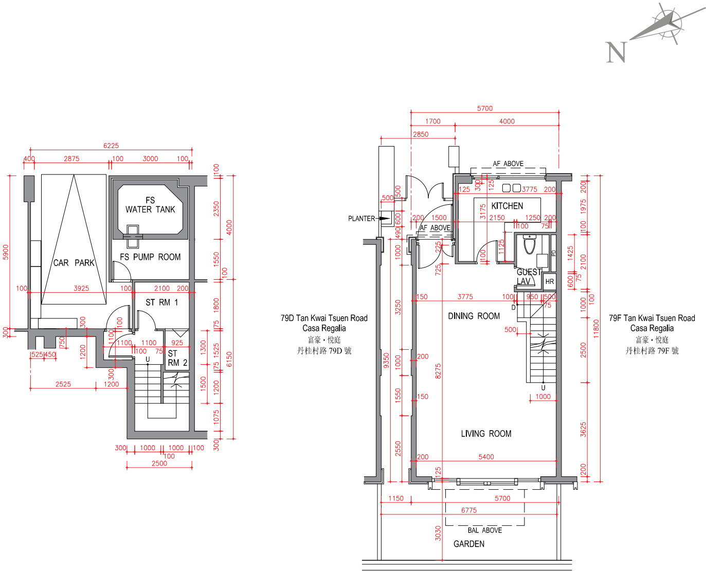
Basement Plan 地庫平面圖
