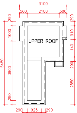
Upper Roof Plan 上層天台平面圖
