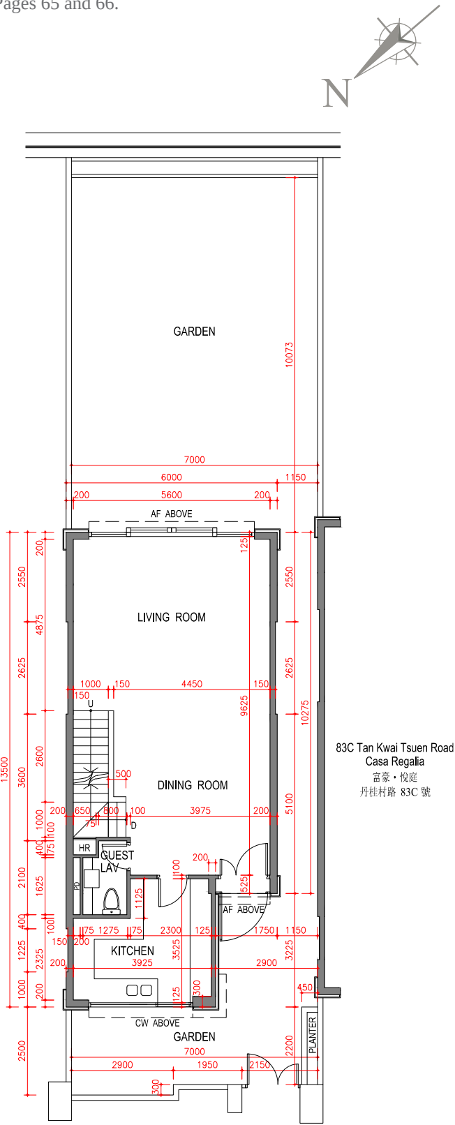
G/F Plan in "as-is" Layout 地面層現狀平面圖
